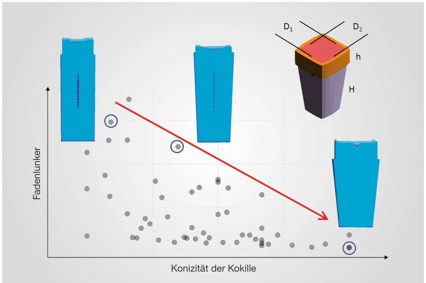
Optimierung der Blockgeometrie zur Vermeidung von Fadenlunkern
