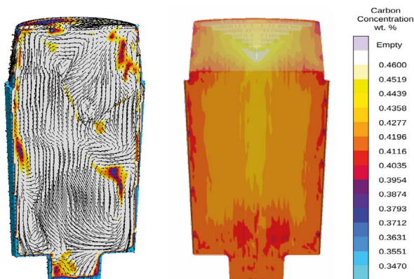
Konvektionsströmung und Bewertung der Produktqualität am Beispiel der Kohlenstoffseigerung
