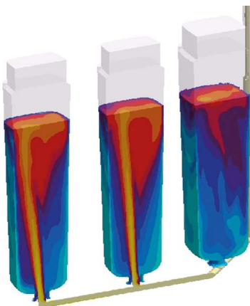
Abguss im Gespann: Simulation der Füllung
