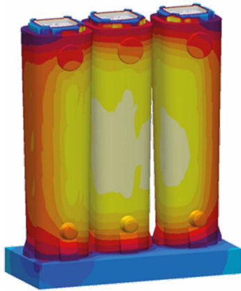
Abguss im Gespann: gleichmäßige Erstarrung gewährleisten
