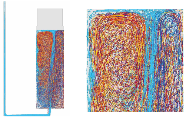
Bewertung des Reinheitsgrades durch Vorhersage von Reoxidationseinschlüssen
