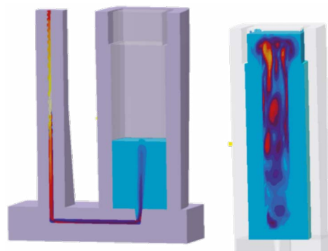
Strömungsgeschwindigkeiten beim Abguss
