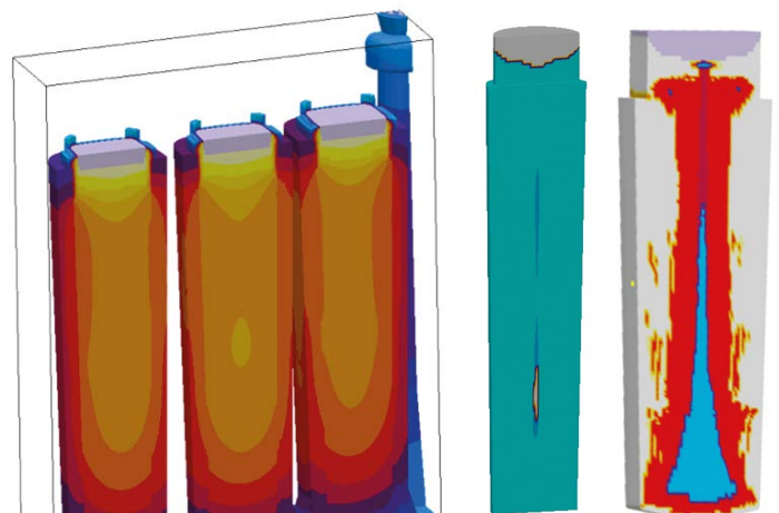
Block- und Kokillentemperaturen im Gespann (links); Porositätsanzeige, CET-Zone (rechts)
