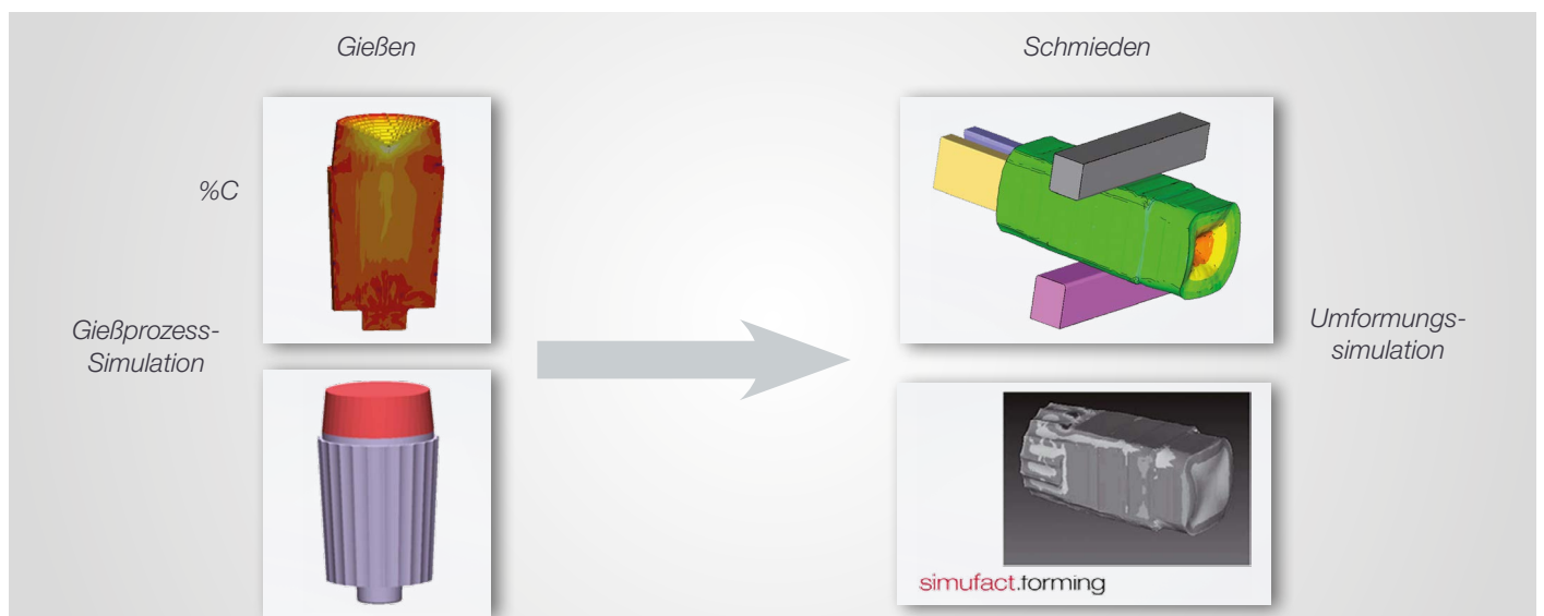
Simulation der durchgängigen Prozesskette – Übertragung von Guseigenschaften auf eine Umformungssimulation
