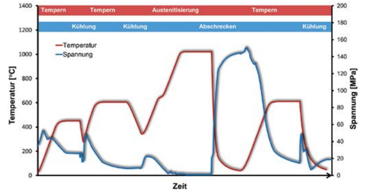
Charakteristisches Temperaturprofil und damit verbundene Spannungsentwicklung während der Wärmebehandlung
