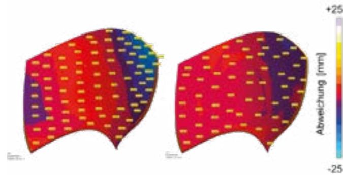
Reduzierung der Verformung durch Vorkompensation nach dem gesamten Herstellungsprozess im Vergleich zur Ausgangssituation (links).
