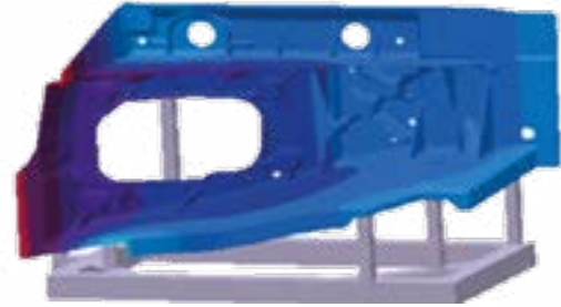
Bewertung verschiedener Gestell-Designs
