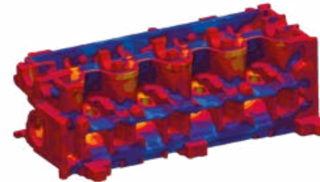
Eigenspannungen in einem Zylinderkopf nach Wärmebehandlung
