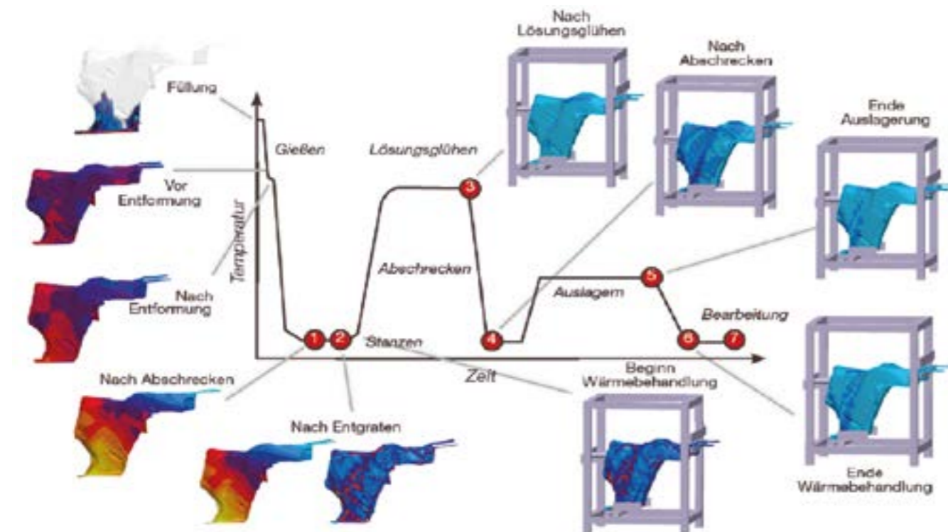
Integrierte Modellierung des Gieß- und Wärmebehandlungsprozesses
