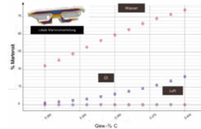
% Martensit in Abhängigkeit von % C und Abschreckmedium
