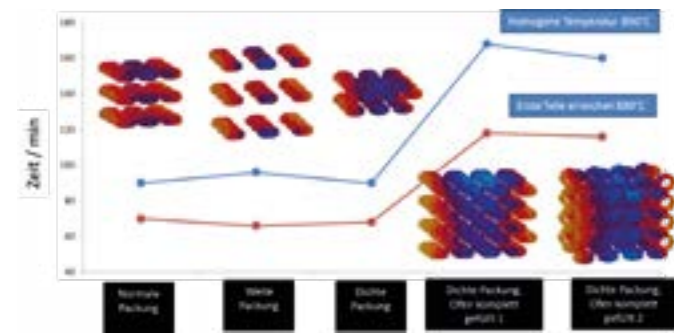
Austenitisierungszeiten für verschiedene Packungen
