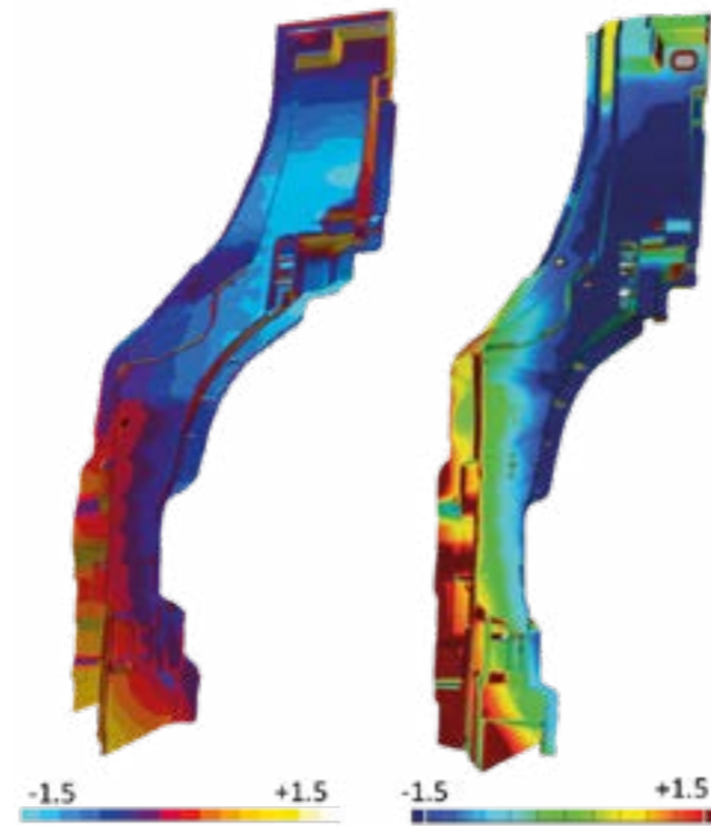
Auswertung des berechneten Verzugs nach der RPS Methode
