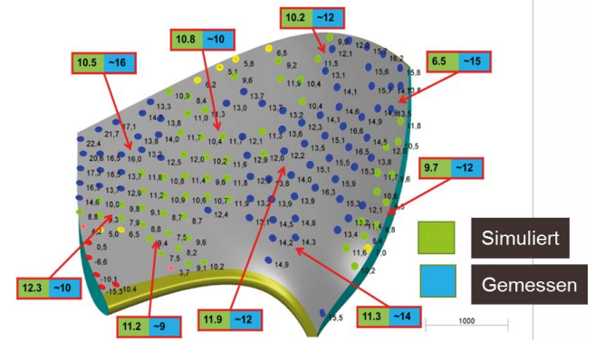
Vergleich von gemessenen und berechneten Verzügen
