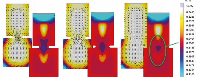
Vorhersage von Seigerungen unterhalb des Speisers
